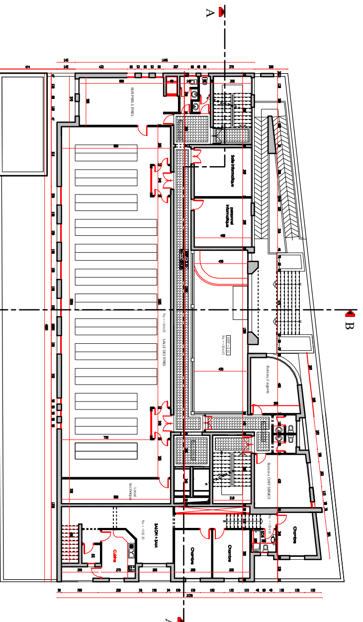
PLAN 1ER ETAGE ECH:1/100
