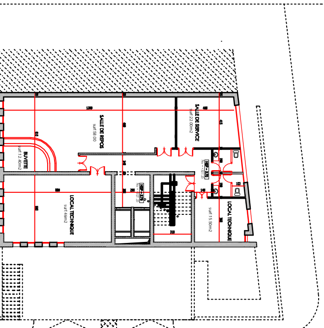
PLAN REZ DE JARDIN ECH : 1/100
